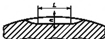
h = (10 \pm 1,5) \% \text{ толщины стенки, но не менее 0,3 мм}
